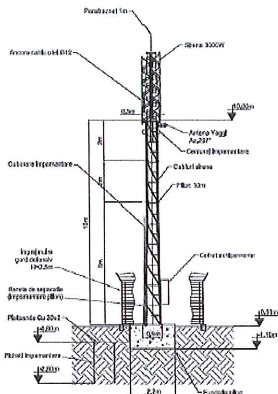
Fig. 4 – Pilon zăbrelelit H=10-30m-elevație
